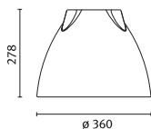
Opta diffuser 36
